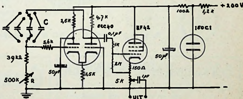
Fig. 1. Principeschema van de vierkantsgolfgenerator. De stabilisatorbuis 150 C1 is niet strikt noodzakelijk. Inplaats van de ECC40 kunnen ook de ECC91 (met kathodeweerstand van 680 Ohm) en 6SN7 (kathodeweerstand 1,2 kOhm) gebruikt worden.
