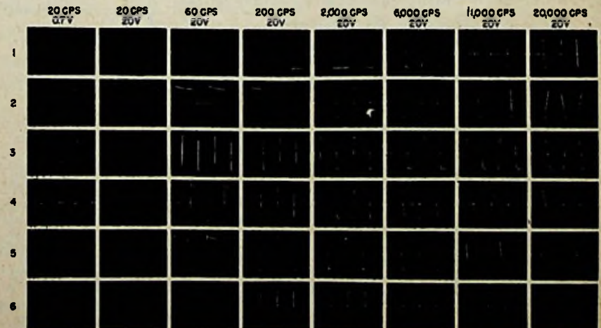
Fig. 3. Vierkantsgolf-analyse aan een aantal bekende uitgangstransformatoren
